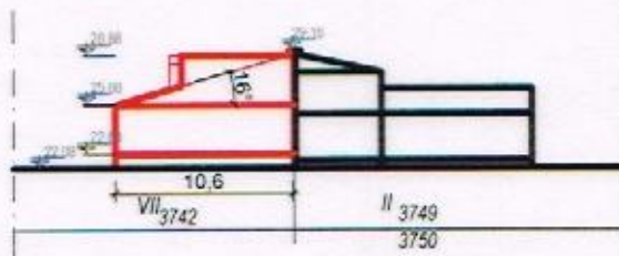
Разрез "а-а" 1:500
