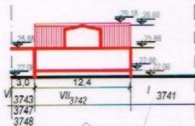
Разрез "б-б" 1:500
